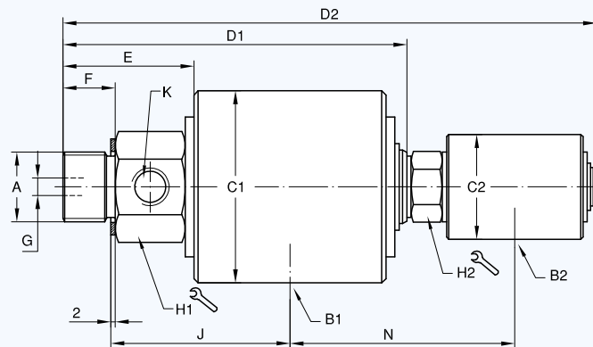
Двухпоточное ротационное соединение (тандем)
